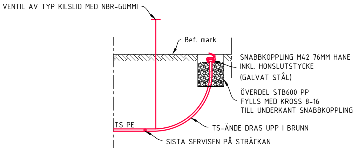
Sektion A-A
